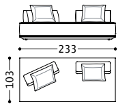
01YK1C6 (1YK1311 + 1YK1CSRT (nr.2) + 1YK1CSH (nr.2))
