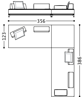
01YK2C2 (1YK2421 + 1YK2431 + 1YK2411 + 1YK2CSRT (nr.4) + 1YK2CSH (nr.2) + 1YK2CBR)
